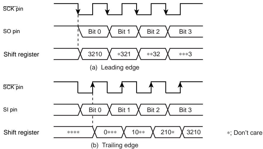
Figure 11-5 Shift edge
