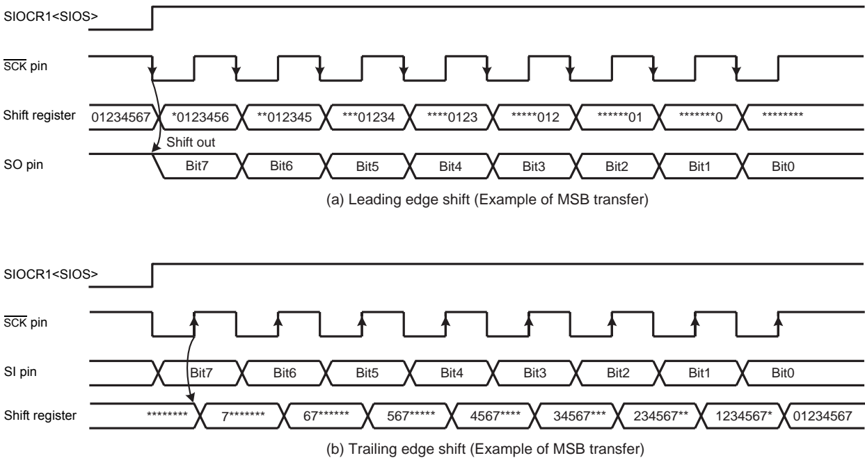
Figure 11-4 Shift Edge
