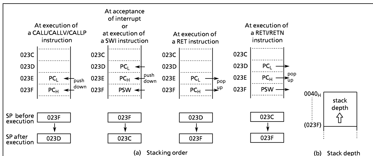
Figure 1-8. Stack
