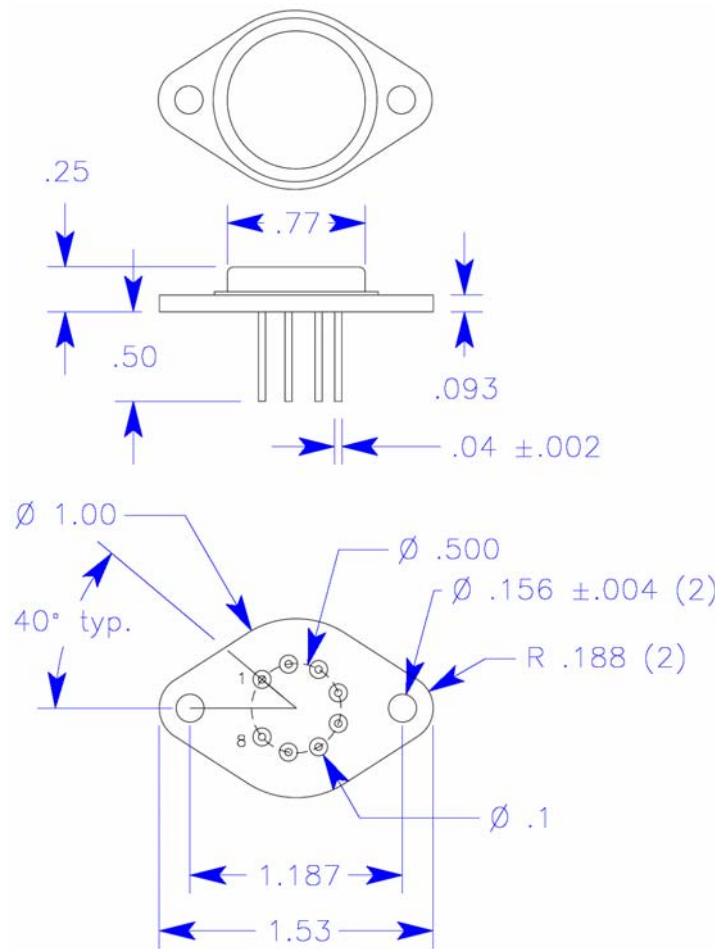
TO3-8 Package
