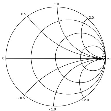
IF Amp Input Impedance (Pin 3) 1. 10.7MHz: 2.2k - j740.8
