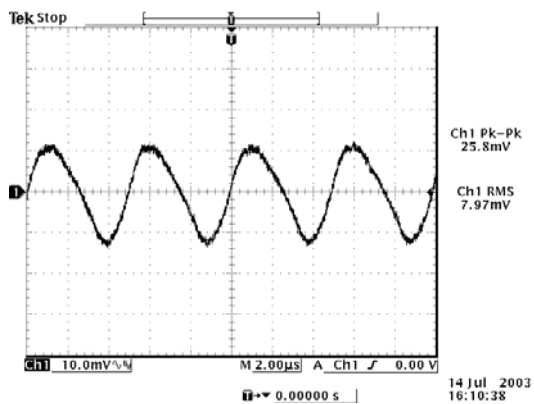
Vin=5 V, Vo=1.5 V
