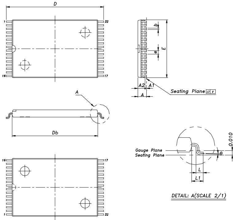
STSOP-32
