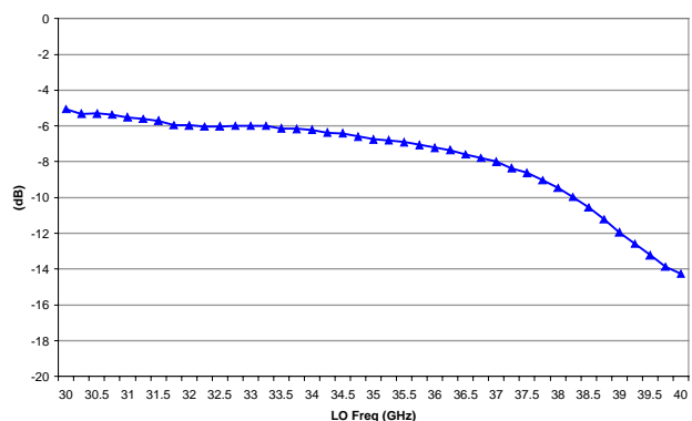
LO Return Loss (dB)
