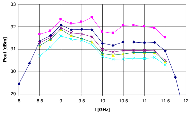
Output power ( V_d=8V , V_{gg}=-5V , P_s=17dBm )
