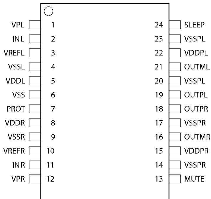
&lt;24 pin SSOP Top View&gt;
