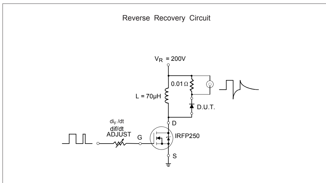
Fig. 11- Reverse Recovery Parameter Test Circuit
