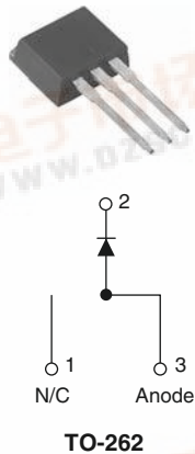
15ETX06-1PbF
