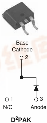
15ETX06SPbF
