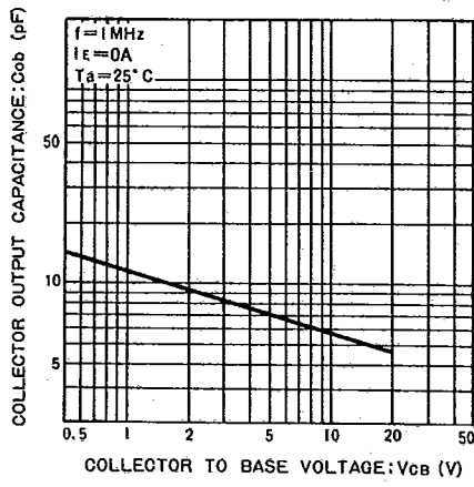
Fig.7 コレクタ出力容量—コレクタ・ベース電圧特性
