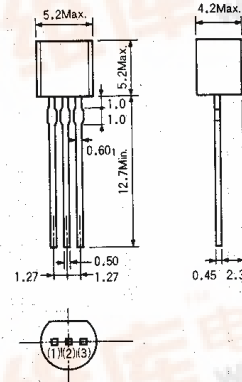
図1 JEDEC:T0-92 EIAJ:SC-43
