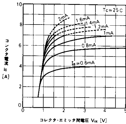
出力特性
