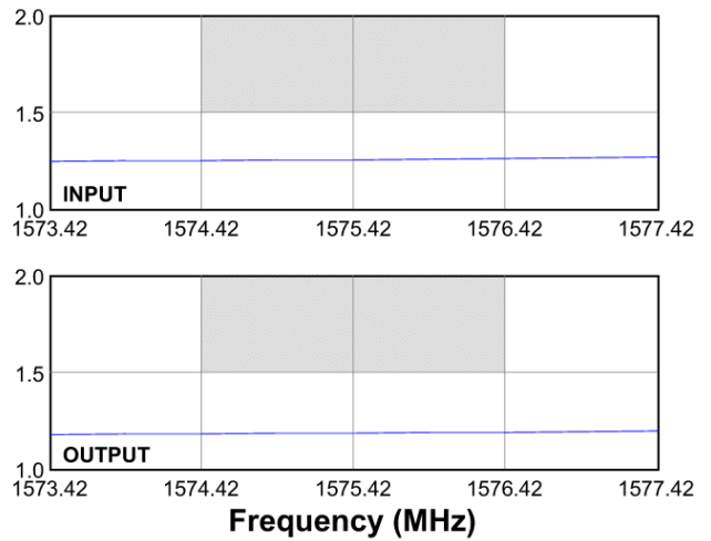
Input/Output VSWR
