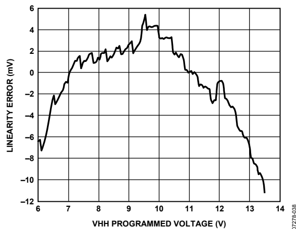
Figure 30. HVOUT VHH Linearity Error
