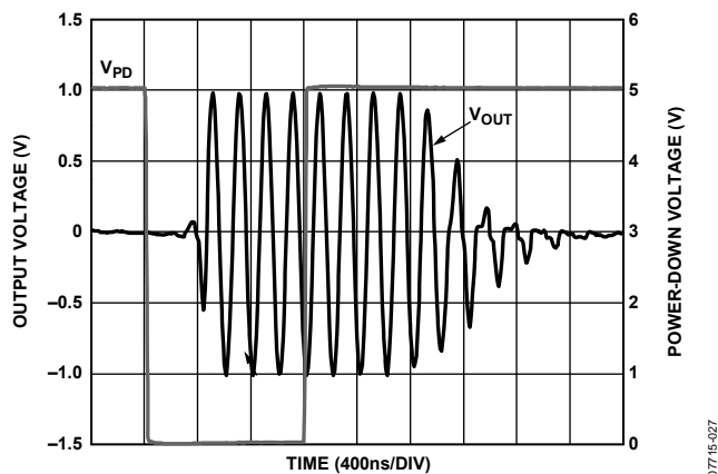
Figure 27. Enable/Power-Down Time
