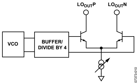
Figure 18. LO Output Section
