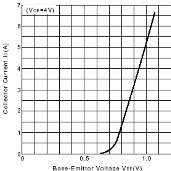
Fig.7 I_c - V_{BE}
