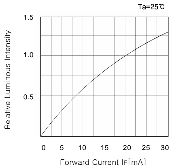
Fig. 2 I_v - I_F
