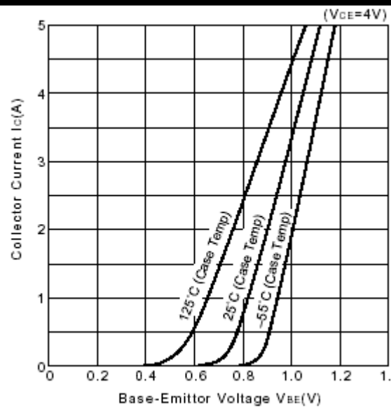
Fig.4 I C -V BE
