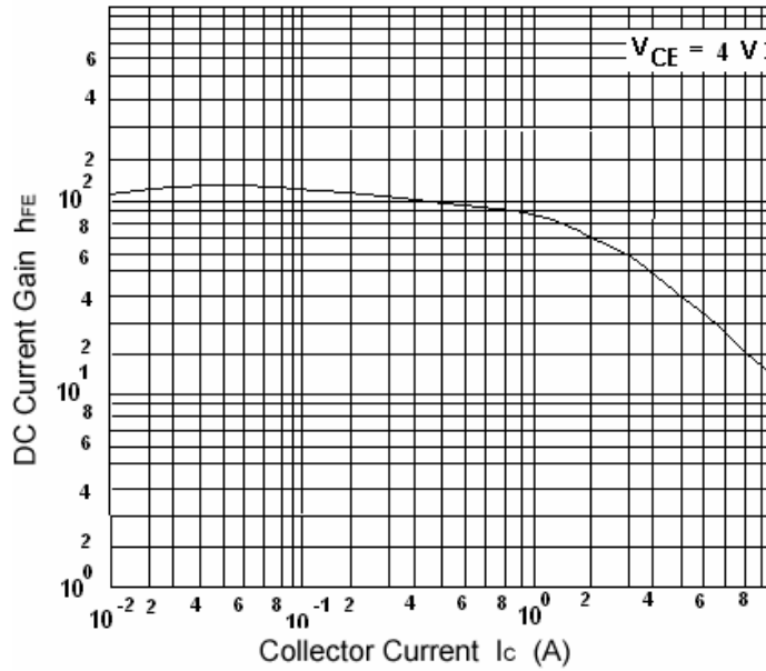
Fig.3 h_{FE} - I_C
