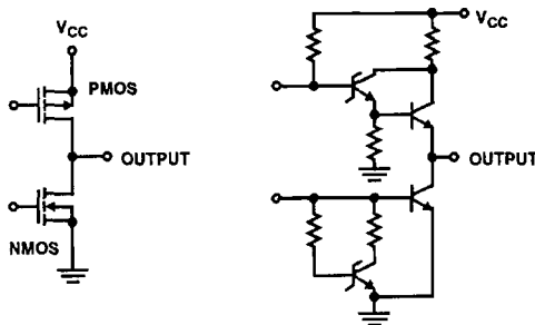
A. CMOS OUTPUT
