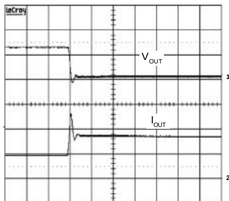
Ch1 : V_{OUT} , 1V/Div, DC Ch2 : I_{OUT} , 2A/Div Time : 50 \mu s /Div
