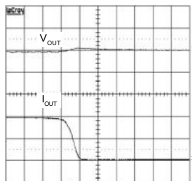
Ch1 : V_{OUT} , 20mV/Div, AC Ch2 : I_{OUT} , 1A/Div Time : 1 \mu s /Div
