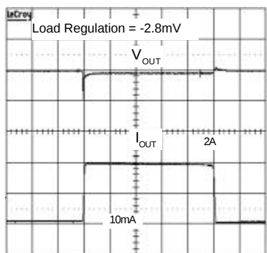
Ch1 : V_{OUT} , 20mV/Div, AC Ch2 : I_{OUT} , 1A/Div Time : 10 \mu s /Div
