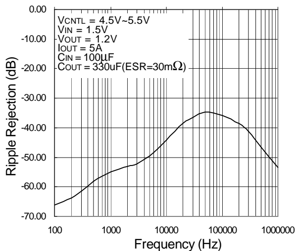
VCNTL PSRR
