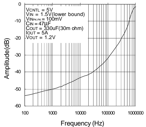
VIN PSRR
