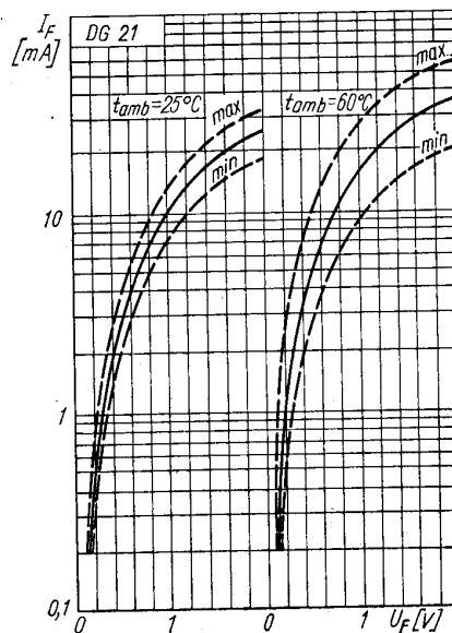
Charakterystyka przewodzenia I_F = f(U_F)
