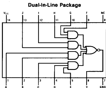
DM54L54 (J) DM74L54 (N)
