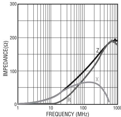
MG 1608- 101Y
