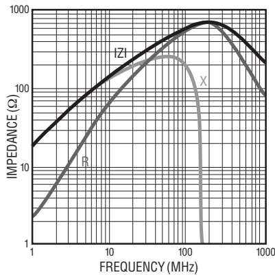
MU 1005- 100Y
