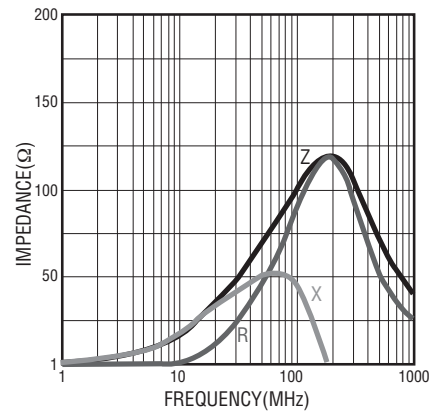
MU 2029- 221Y
