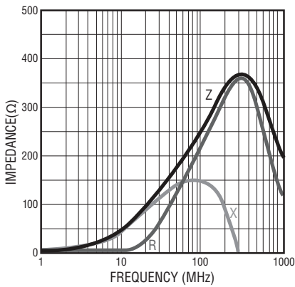
MU 1005- 471Y
