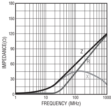
MG 2029- 121Y
