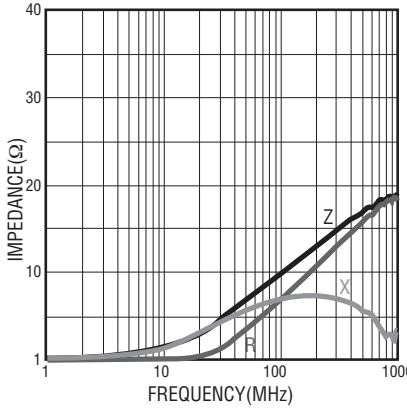
MU 2029- 600Y
