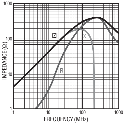
MU 1608- 300Y
