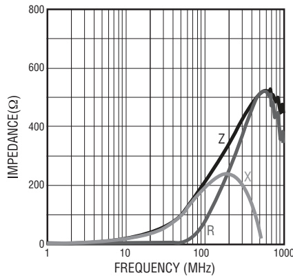
MU 1005- 601Y
