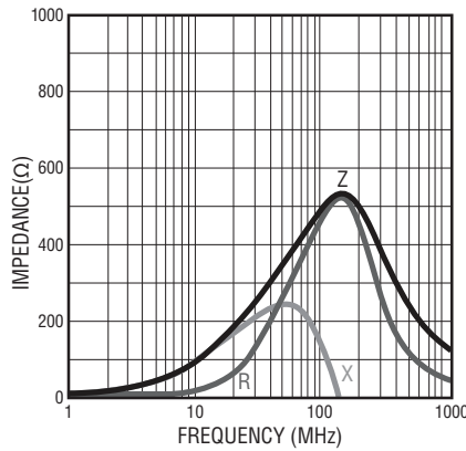
MG 1608- 400Y
