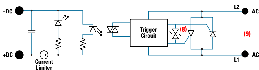
Diagram: HAC DC control
