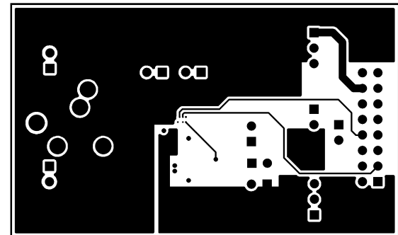
Figure 41. Bottom Layer
