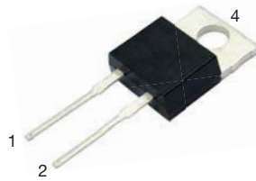
2L TO-220AC
