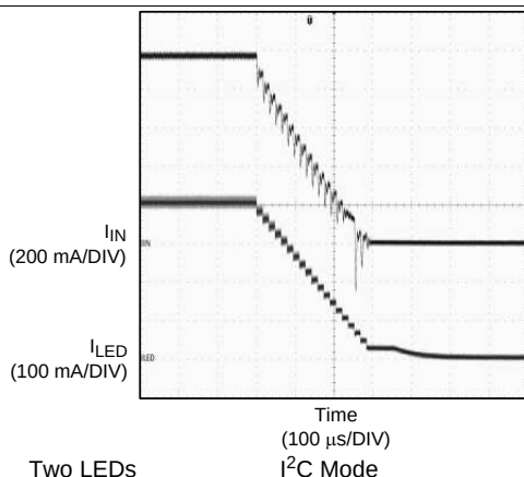
Figure 27. Ramp-Down (Zoom)
