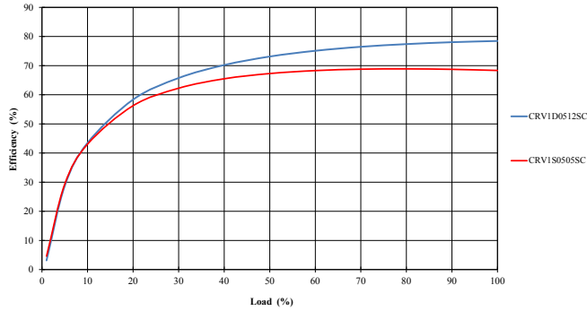
5V Inputs
