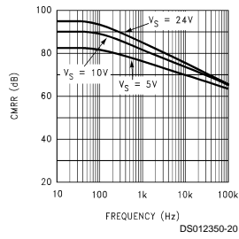
CMRR
