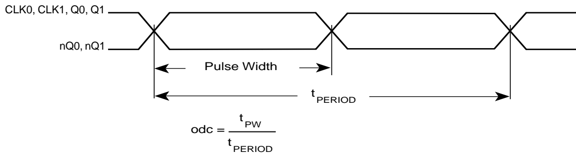
FIGURE 5 - odc & t_{PERIOD}
