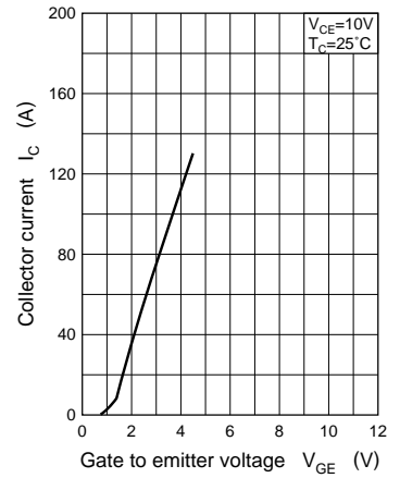
I_C - V_{GE}
