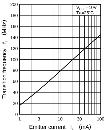
f_T - I_E
