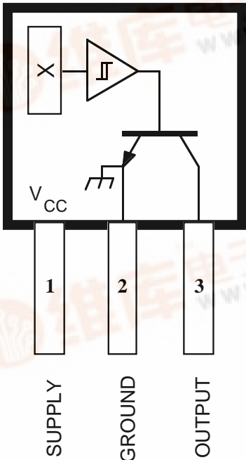
Dwg. PH-003A
