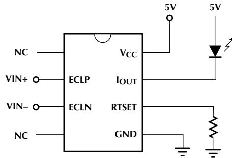
a) I_{OUT} = 75mA
