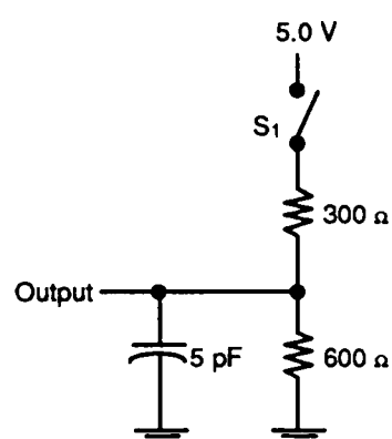
B. Output Load for TGVQZ
