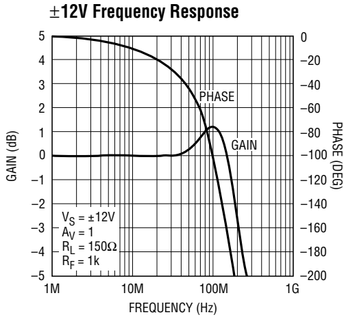
LT1253/54 • TPC10
