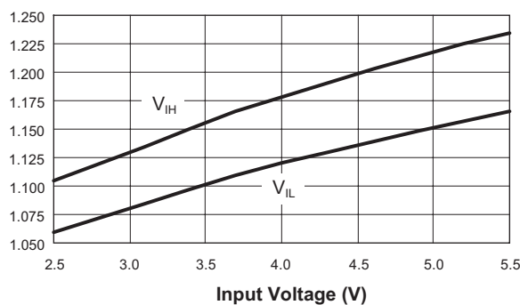
LDO ENLDO vs. V_{IN}
