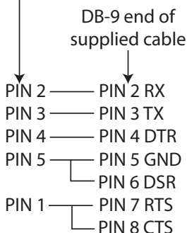
DIN to DB-9 Cable
