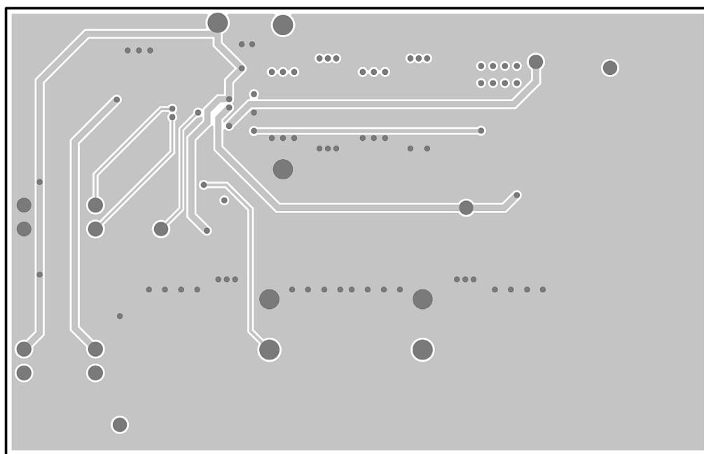
FIGURE 22. Bottom Layer
