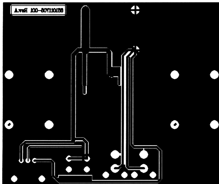
Bottom Layer (2) LM4843MH
