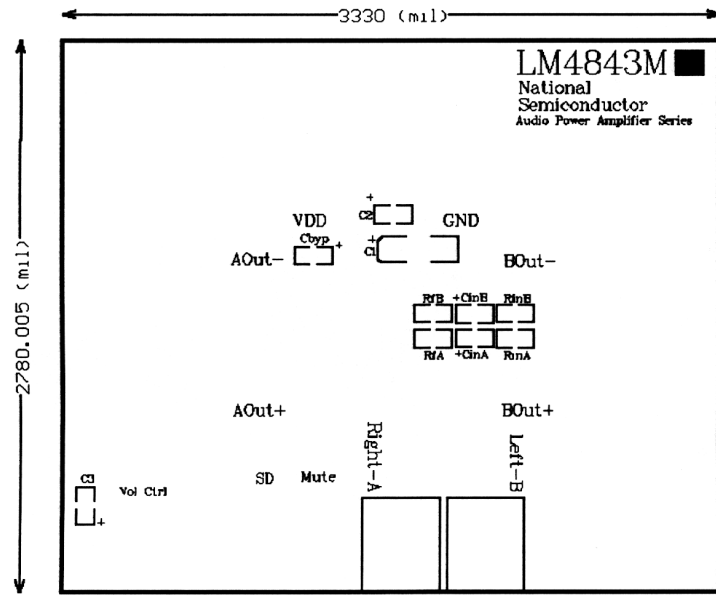
Top Layer SilkScreen
