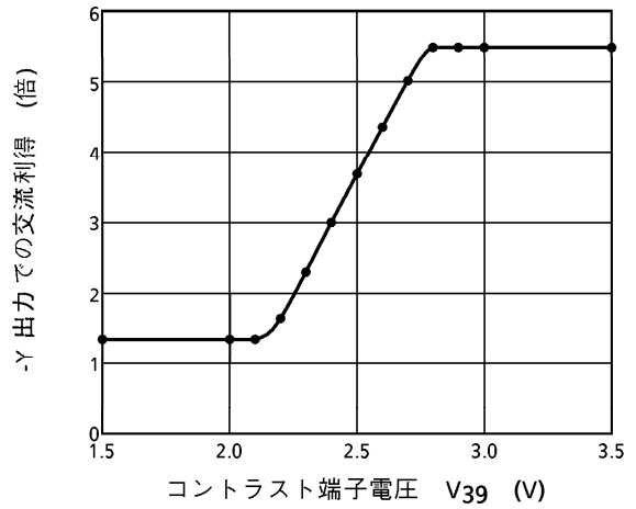
コントラストコントロール特性
