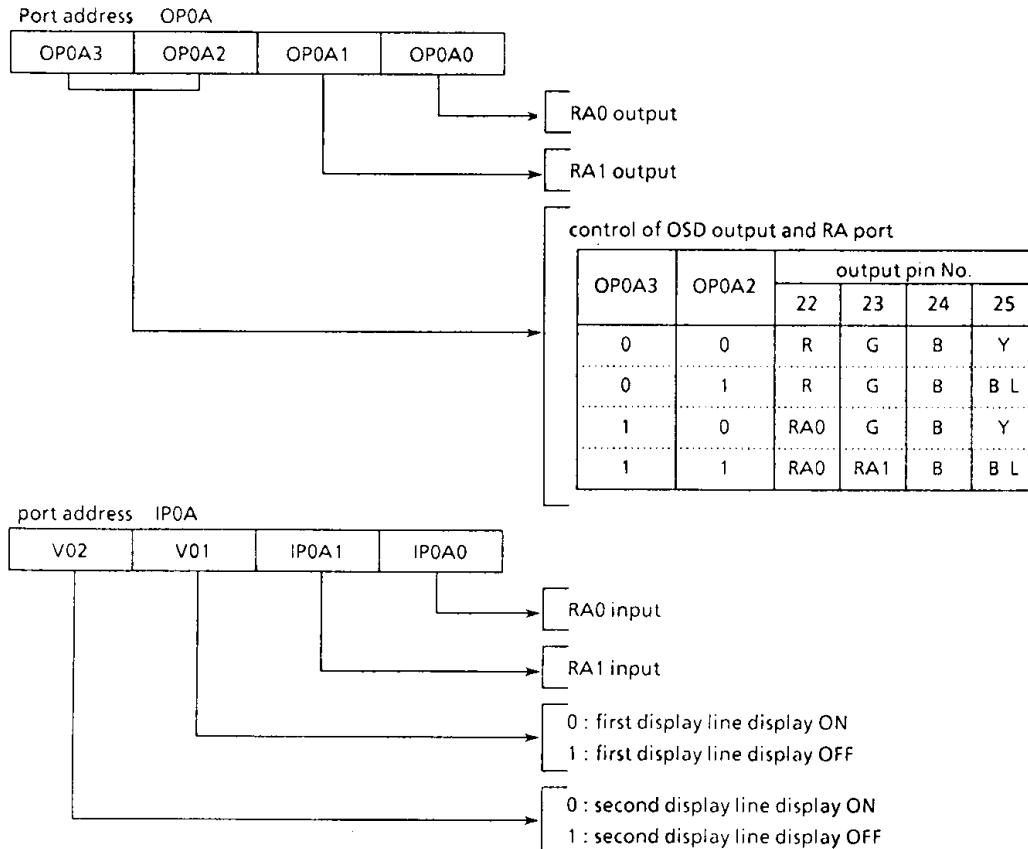
Figure 3-8. Port RA
