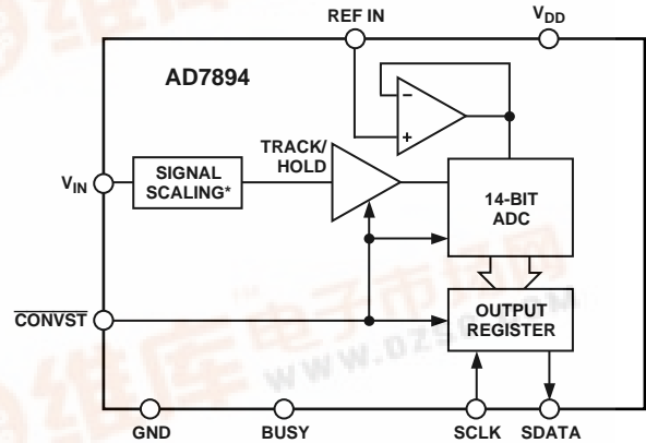
*AD7894-10, AD7894-3
