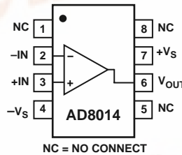
SOIC-8 (R)
